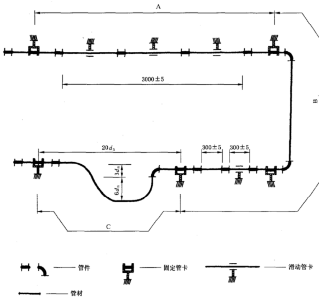
图 1 试验装配图
